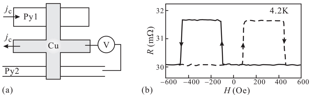
図 7.2 (a) スピン注入効果の非局所測定配置. 電流 j_c は Cu のクロス点を通して左へ抜けるが, Py1 より注入されたスピン流は Py2 へ達して界面にスピン蓄積することで \mu_0 のステップを引き起こし, 電圧 V として検出される. (b) 測定された非局所抵抗. スピンパルプ的磁気抵抗は, Py1 と Py2 の形状の違いによる保磁力差によるもの. データは文献 [2] より.
