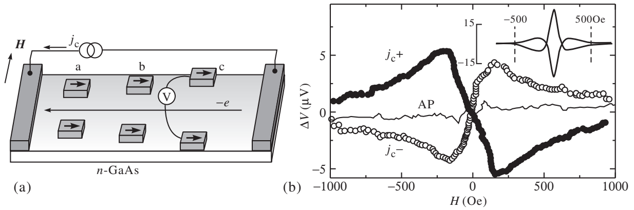
図 7.6 (a) n 型 GaAs 試料の電極配置. 電流に垂直に対向した Fe 電極で, 試料端のスピンの蓄積を検出する. (b) 試料端から 2\mu\text{m} にある電極でのスピンの蓄積信号. 電流密度は 5.7 \times 10^3 \text{ A/cm}^2 . 黒丸白丸は平行磁化配置に電流の向きを反転した結果, 実線は反平行磁化配置の結果. 挿入図は, 電極間の Hanle 効果測定. 温度は 30\text{K} .
