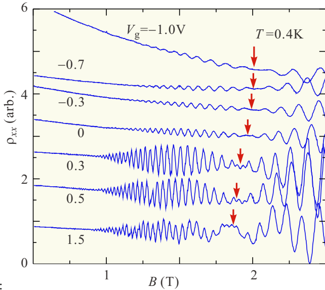
図 7.5 \text{In}_{0.53}\text{Ga}_{0.47}\text{As} 量子井戸中の 2 次元電子系で SdH 振動を測定したもの. 2 次元電子系表面のゲート電極に加える電圧 V_g を変化させている. 矢印はビートの谷の位置を示した. [9] より.
