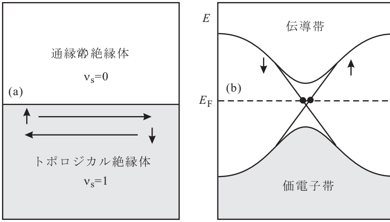
図 7.7 トポジカル絶縁体概念図. (a) y < 0 を 2 次元トポジカル絶縁体が占め、ヘリカル端状態が 1 対生じている. 真空側は通常の絶縁体. 端状態の数に対応してトポジカル絶縁体側のスピンのチャーン数は 1. (b) エネルギー図. 線形分散を持つヘリカル端状態が生じている [10].
