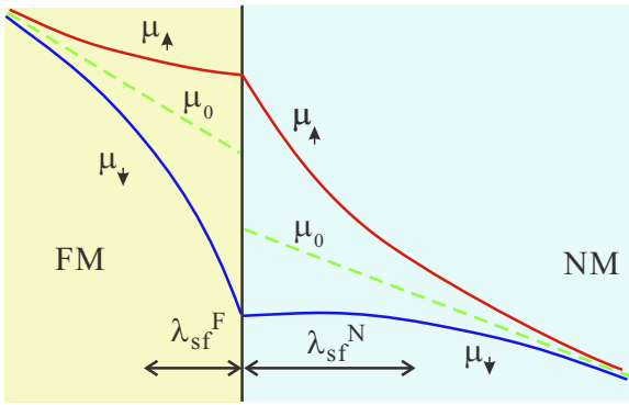
図 7.1 FM-NM 界面に FM 側から電子が流れるような電流の下でのスピン依存化学ポテンシャルの空間変化模式図.
