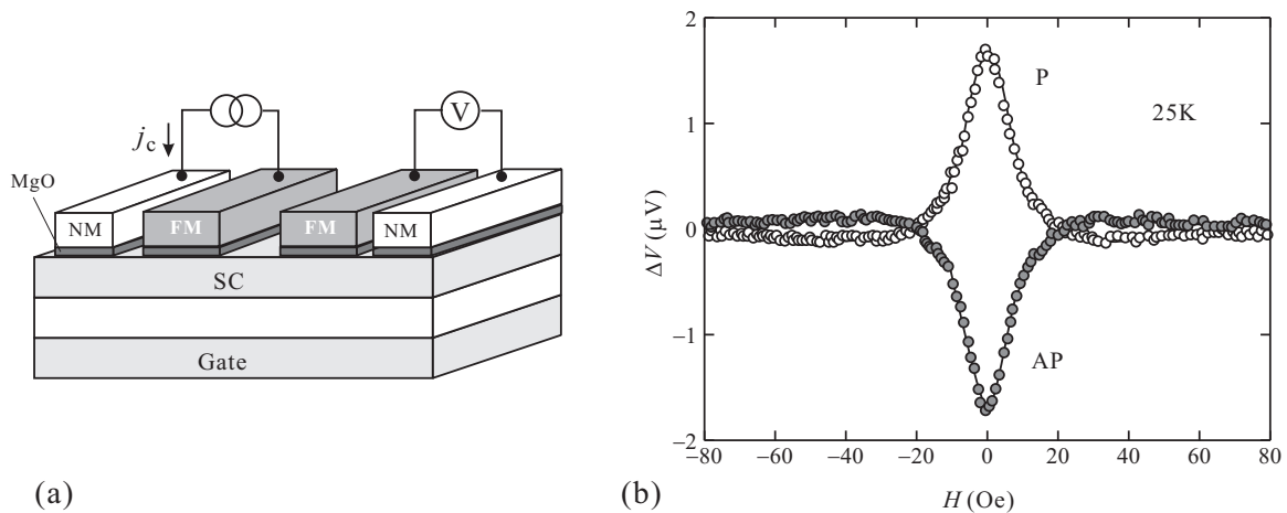
図 7.3 (a) 半導体 (SC) へのスピン注入を 4 端子非局所効果で検出するための電極配置。左の強磁性体 (FM) と常磁性体 (NM) 間に電流 j_c を流すことで、スピン流は右方向へも流れ、右の FM 電極と NM 電極に生じる電気化学ポテンシャル (電位) 差として検出される。注入効率を上げるため、MgO などの絶縁体障壁が用いられる。(b) 左と類似の構造で Si にスピン注入して面垂直磁場によってスピン歳差運動を生じさせて観測された Hanle 信号。文献 [3] より。
