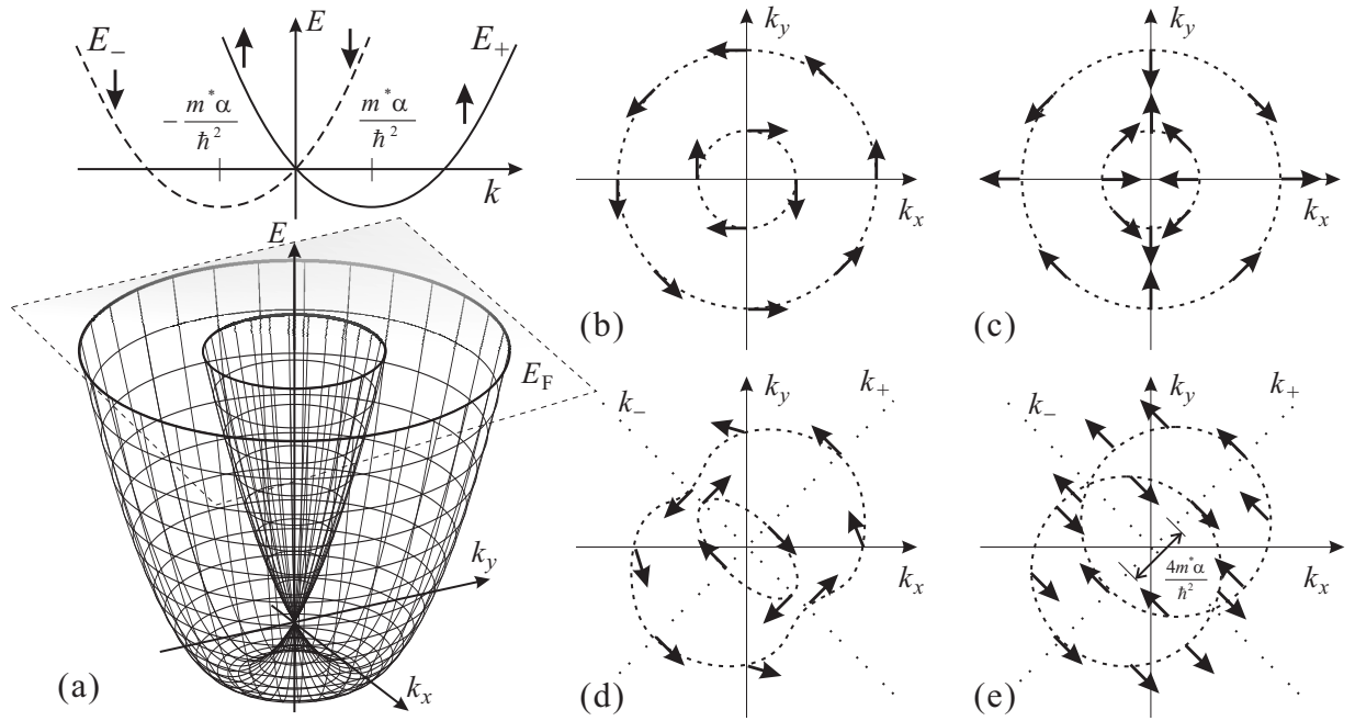
図 7.4 (a) 上: ラシュバ相互作用がある場合のエネルギー分散 (7.20) を描いたもの. +\pi/2 のスピンを上向きとして描いている. 下: k_x - k_y 平面上にエネルギー分散を 3 次元的に描くとこのワイヤフレーム表示のようになる. (b) 以降の図は, E_F の面での切り口を描いている. (b) \beta = 0 (ラシュバ模型) の場合の, 2 つのフェルミ円 (短い破線) 上でのスピンの向き. (c) \alpha = 0 (ドレッシェルハウス模型) の場合. (d) \alpha, \beta が有限で, \alpha \neq \beta の場合. (e) \alpha = \beta の場合.
